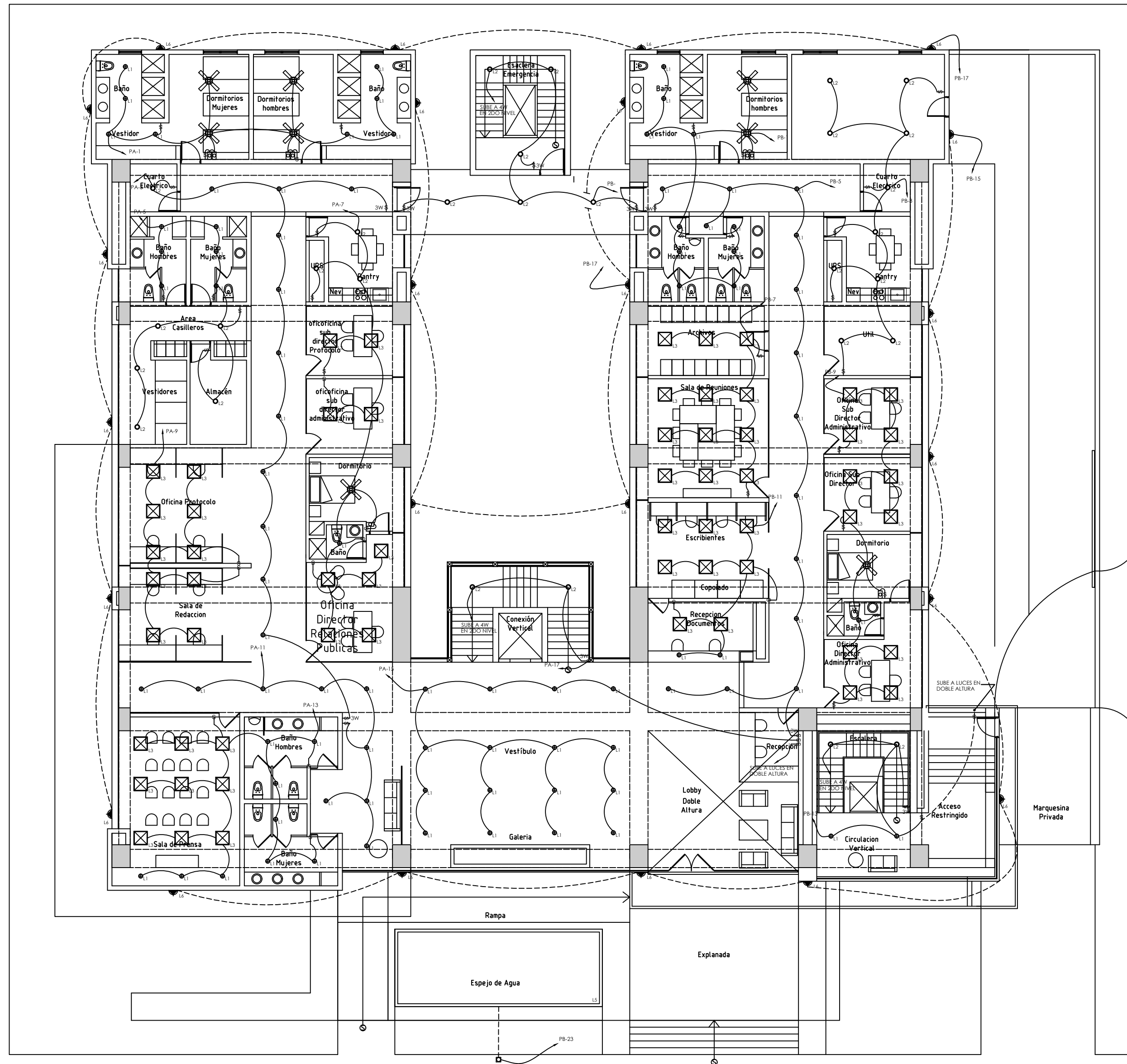
1 E-1 PLANTA ILUMINACION 1ER NIVEL
